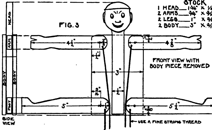
STRING JACK
